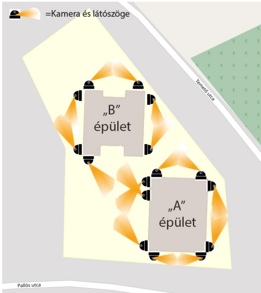
1. ábra A Jókai Mór Református Magyar-Angol Két Tanítási Nyelvű Általános Iskola, AMI és Óvoda iskolai belső udvarának sematikus rajza a kültéri megfigyelőegységekkel és látószögeikkel. Térkép adatforrás: © OpenStreetMap közreműködők ; https://www.openstreetmap.org/copyright ; Licenc: CC BY-SA
