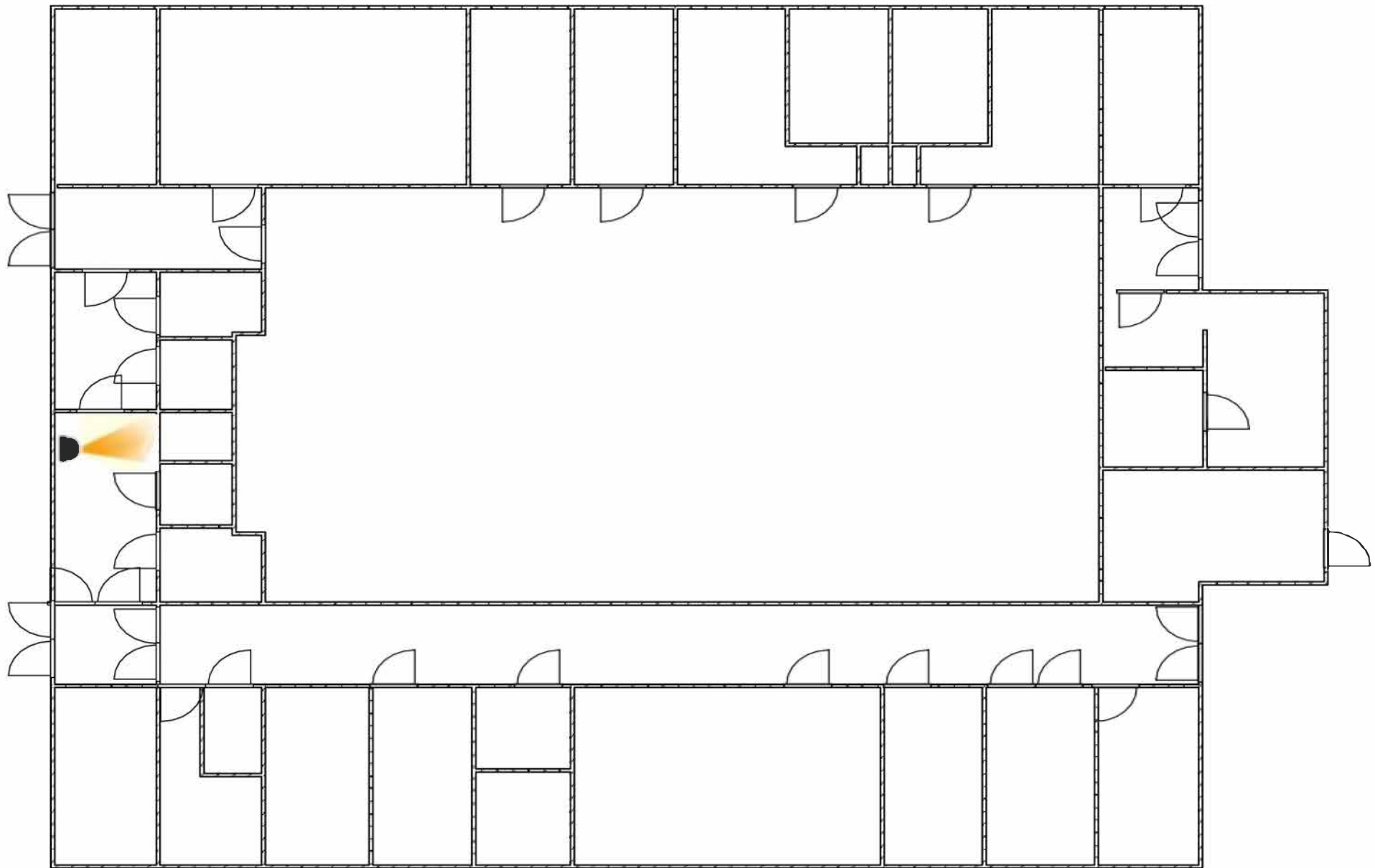
3. ábra A Jókai Mór Református Magyar-Angol Két Tanítási Nyelvű Általános Iskola, AMI és Óvoda „B” épületének földszinti alaprajza a megfigyelőegységekkel és látószögeikkel
